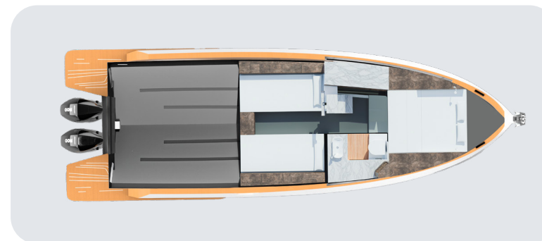
Distribución interior fueraborda.
